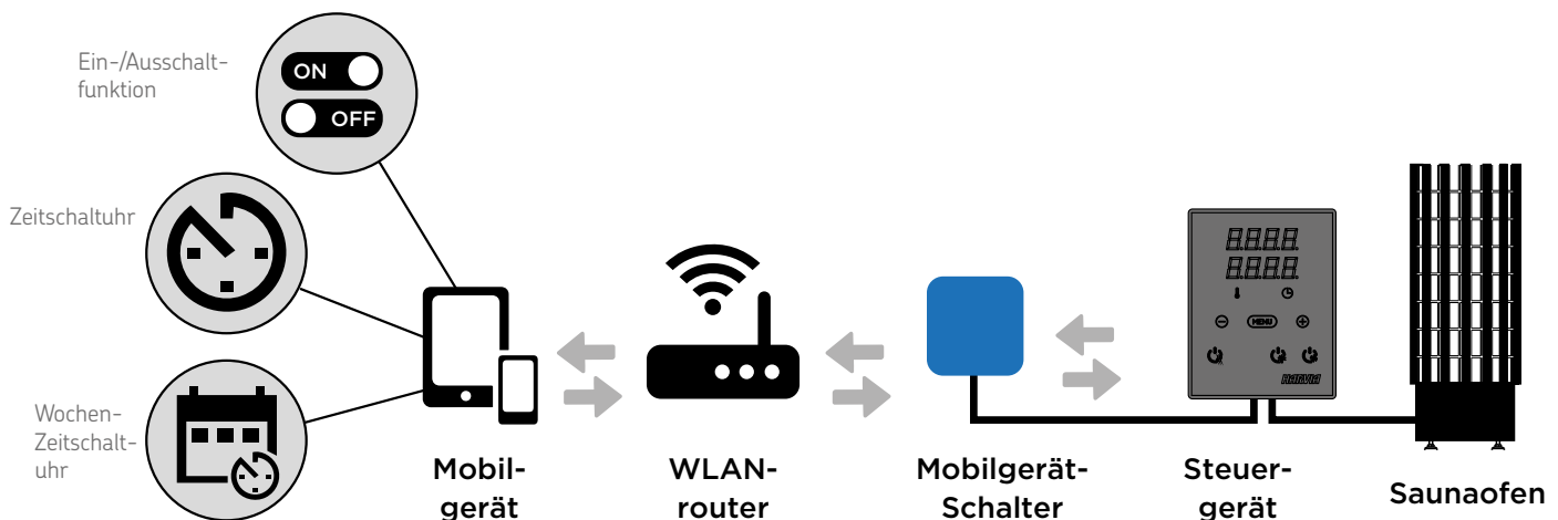
Mobilgerät-Schalter FS-SY
